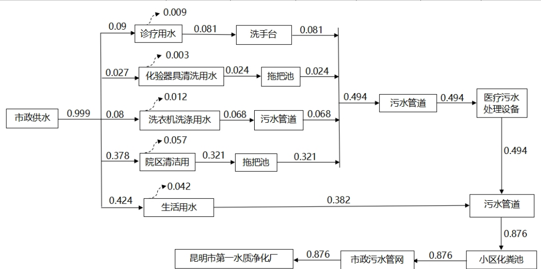
图 2-1 项目运营期水量平衡图 (m 3 /d)
