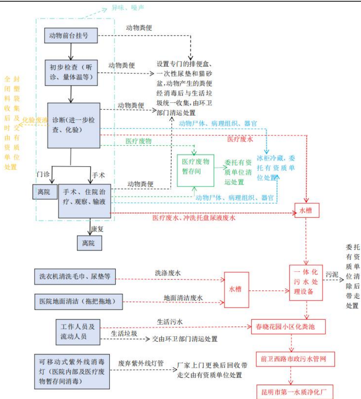
图 2-2 运营期工艺流程及产污节点图
