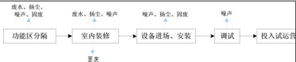
图 2-1 项目施工期工艺流程及产污节点图
