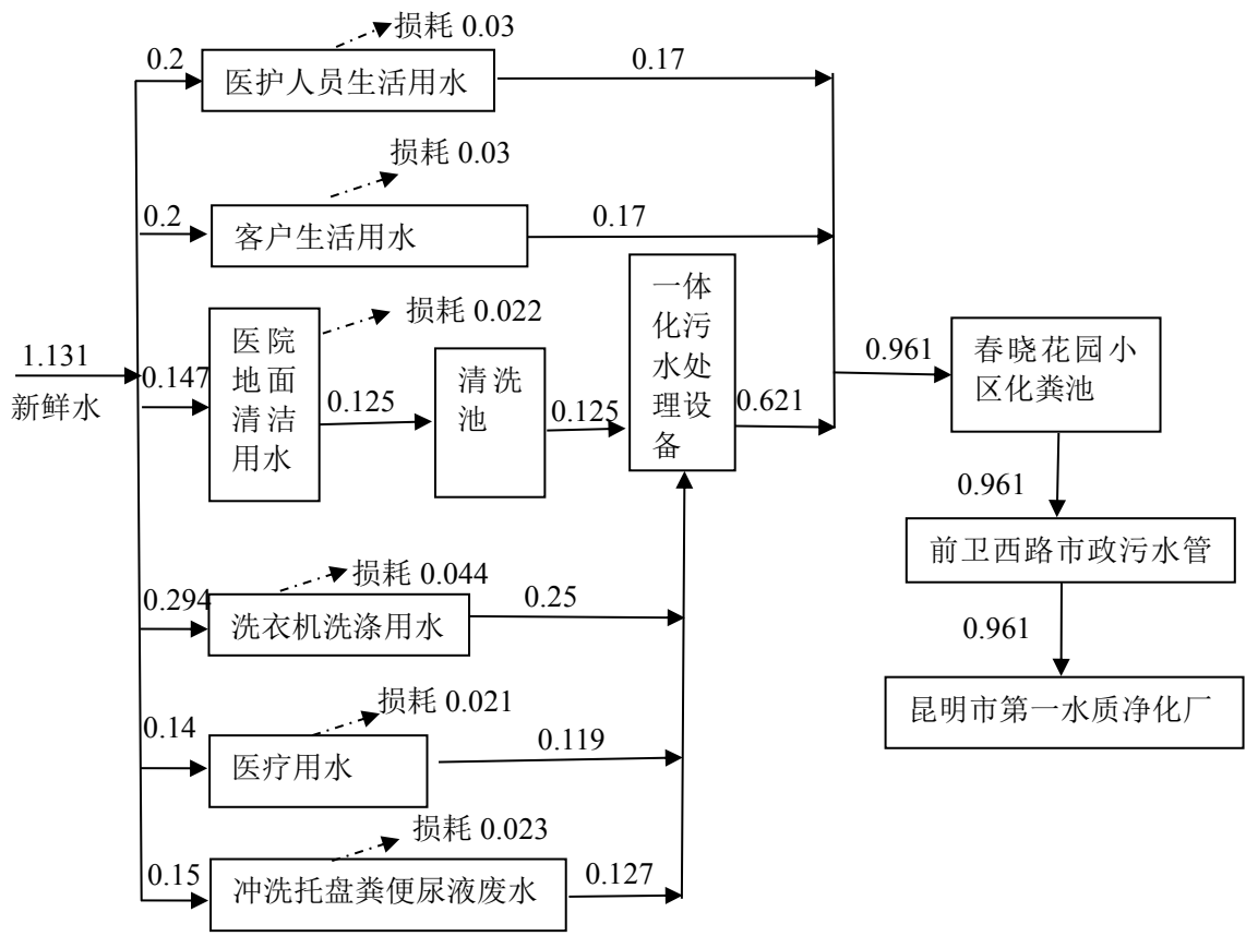
图 4-1 项目水平衡图 单位：m³/d
