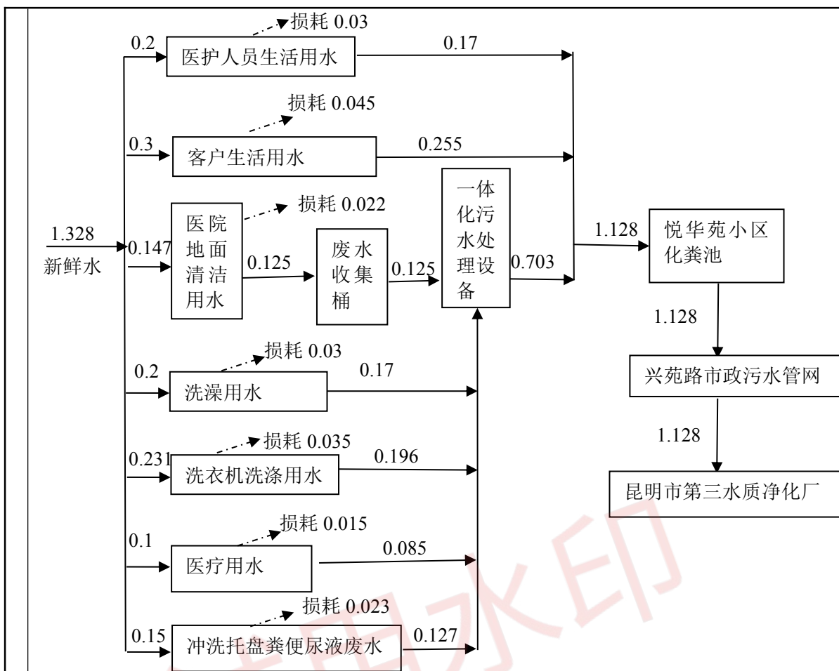
图 4-1 项目水平衡图 单位: \text{m}^3/\text{d}
