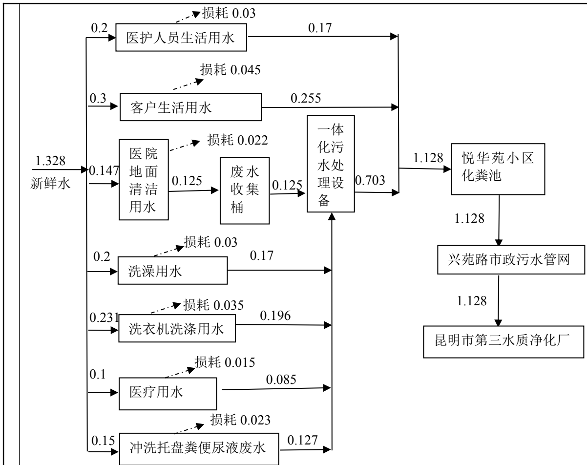
图 4-1 项目水平衡图 单位: m 3 /d
