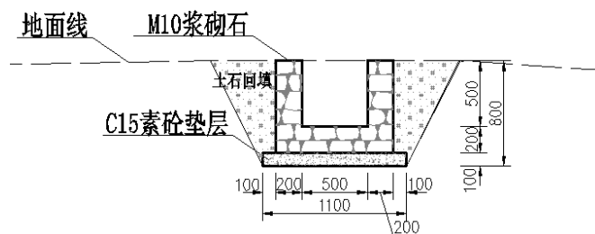
图 2-1 排水沟断面示意图
